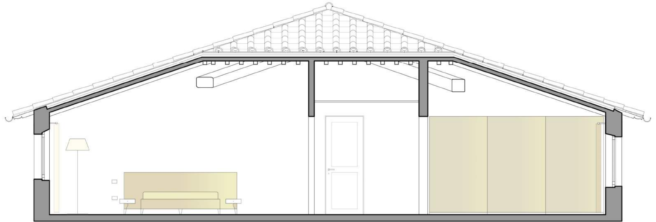
PROSPETTO
