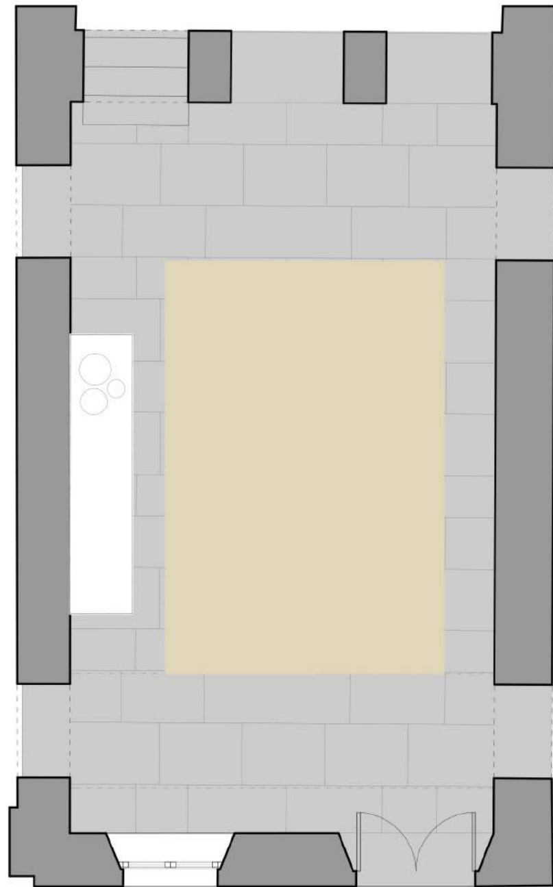
PIANTA scala 1:50
